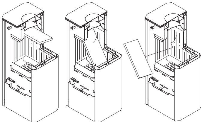
41. Kolejność demontażu oraz wymiany deflektora i wyłożenia acumotte – ENYO The procedure for the baffle and Acumotte lining disassembly and replacement – ENYO
