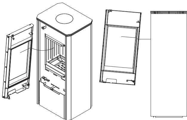
41. Kolejność demontażu oraz wymiany deflektora i wyłożenia acumotte – ENYO The procedure for the baffle and Acumotte lining disassembly and replacement – ENYO
